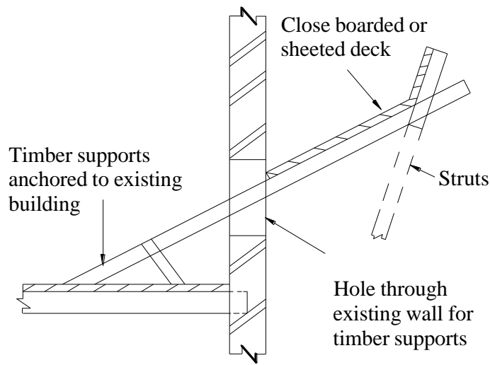
Fig 2.5b Fan hoarding
